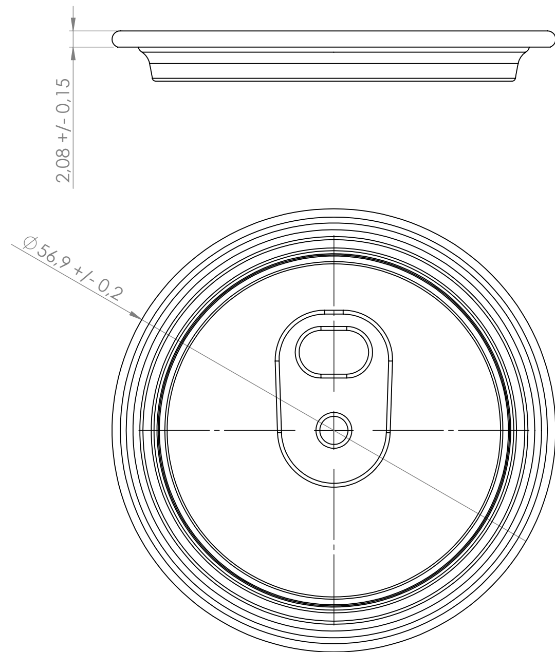
CDL Ø50 (200) LOE
